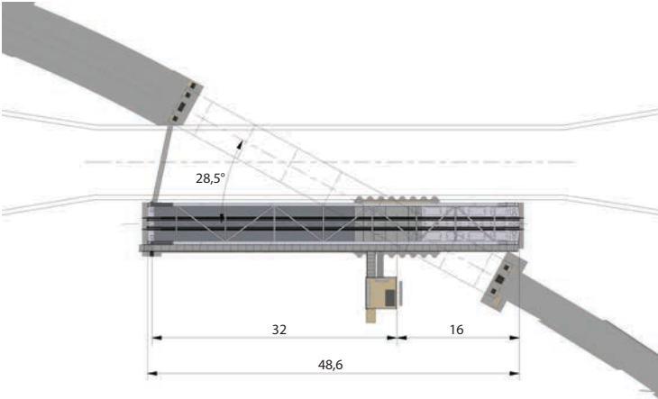
2. Aggregaat en besturingskasten staan buiten de pijler.
